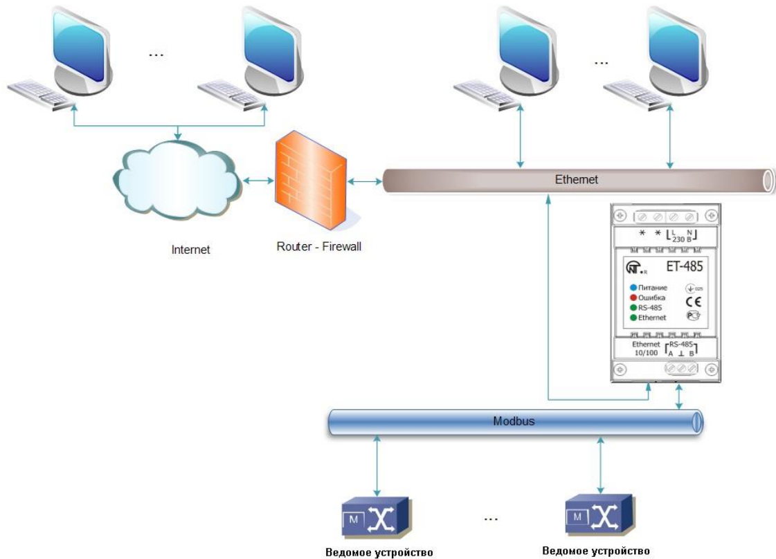
Рисунок В.1 – Доступ к сети RS-485 (Modbus RTU/ASCII) по сети Ethernet (Modbus TCP)
