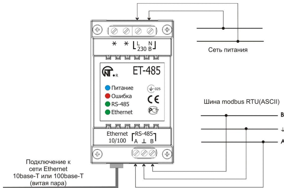
Рисунок 4 – Схема подключения прибора
