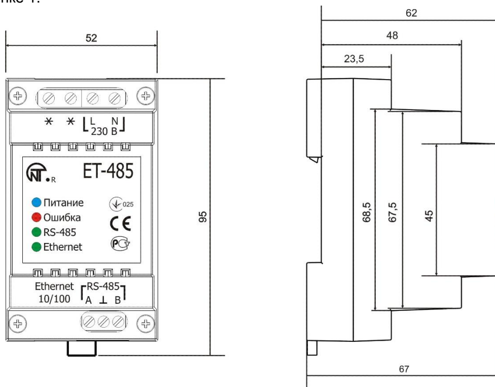
Рисунок 1 – Габаритные размеры прибора
